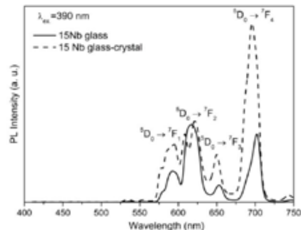
Фигура 1. Сравнение на луминесцентните спектри на стъкло със състав 35\text{WO}_3\cdot 24\text{La}_2\text{O}_3\cdot 25\text{B}_2\text{O}_3\cdot 15\text{Nb}_2\text{O}_5\cdot 1\text{Eu}_2\text{O}_3 (mol %) и получения стъклокристален образец (съдържащ \text{LaWBO}_6 ) след нагряване на същия състав стъкло (дължина на вълна на възбуждане \lambda_{\text{ex}}=390 nm)
