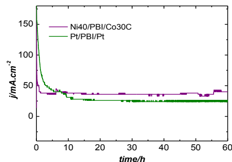
Фигура 1. Потенциостатични криви, МЕП5 с Ni40 катод и Co30 анод и МЕП2 с Pt катод и Pt анод, E = 2 V
