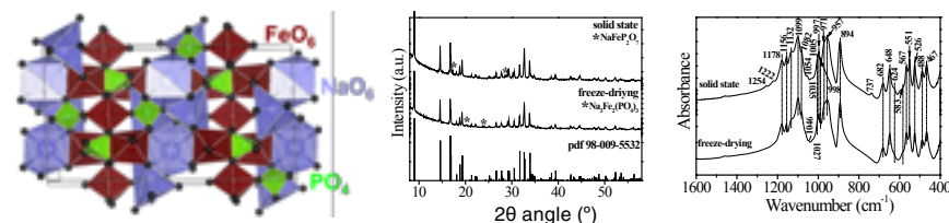
Фигура 1. Кристална структура (а); Рентгенофазов анализ (б) и ИЧ спектър (в) на \text{Na}_3\text{Fe}_3(\text{PO}_4)_4 получен чрез лиофилизация и твърдофазен синтез.
