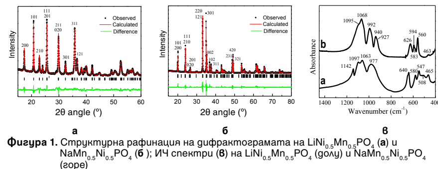
Фигура 1. Структурна рафинация на дифрактограмата на \text{LiNi}_{0.5}\text{Mn}_{0.5}\text{PO}_4 (а) и \text{NaNi}_{0.5}\text{Mn}_{0.5}\text{PO}_4 (б); ИЧ спектри (в) на \text{LiNi}_{0.5}\text{Mn}_{0.5}\text{PO}_4 (долу) и \text{NaNi}_{0.5}\text{Mn}_{0.5}\text{PO}_4 (горе)
