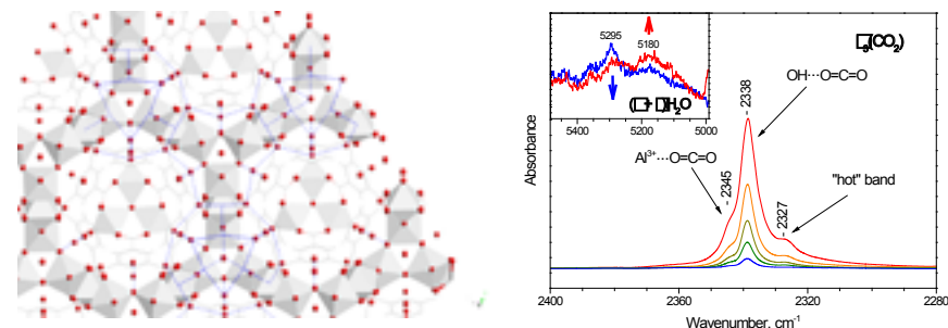
Фигура 1. Отляво: Структура на MIL-96(Al). Отдясно: ИЧ спектри на CO 2 , адсорбиран върху MIL-96(Al). Малкото каре показва, че CO 2 измества координираната H 2 O.
