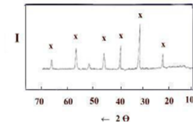
Фигура 1. РФА на керамиката, синтезирана при 1300^\circ C , x-BaTiO_3 .
