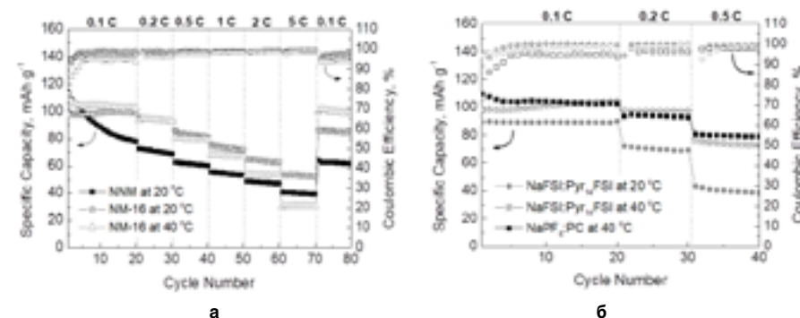
Фигура 1. Способност за работа при различни скорости на заряд и разряд на (а) изхожен оксид (20 °C) и заместен (20 и 40 °C) в присъствие на електролит \text{NaPF}_6\text{:PC} и (б) заместен оксид в присъствие на електролит \text{NaPF}_6\text{:PC} (20 oC) и \text{NaFSI:Pyr}_{14}\text{FSI} (20 и 40 oC) и в потенциални граници 2.0 – 4.3 V.
