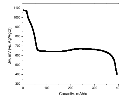
Фигура 2. Електрохимична разрядна крива на композита Mg_{2.1}Ni_{0.7}V_{0.3} – 5 мас. %, използван като отрицателен електрод в Ni/MH батерия.
