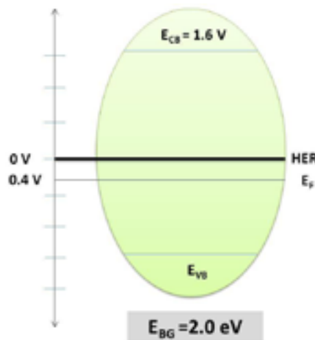
Фигура 1. Енергийна зонава диаграма на филми от \text{FeS} отложени върху FTO, за 5 min, E=-0.8 \text{ V} (vs.RHE), T=50^\circ \text{C}
