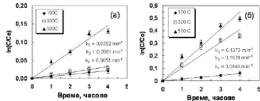
Фигура 2. Зависимост между натурален логаритъм от концентрационното отношение и времето на облъчване за разграждане на (а) Парацетамол и (б) Хлорамфеникол използвайки ZnO филми като фотокатализатори.
