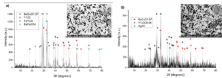
Фигура 1. XRD рентгенограми и SEM микрографии на: а) \text{Y134} + 0.20 тегл.% \text{Fe}_3\text{O}_4 , б) \text{Y134} + 0.20 тегл. % \text{Ag}_2\text{O} .
