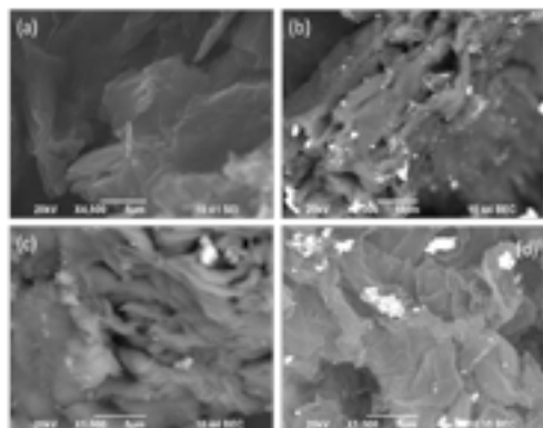
Фигура 1. SEM изображения (a) RGO, (b) RGO/Ag, (c) RGO/Cu, (d) RGO/Cu-Ag.
