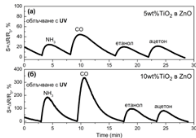
Фигура Отклик (S) на нанокompозитен сензорен елемент, формиран чрез лазерна аблация на: (а) 5 wt % \text{TiO}_2 в ZnO и (б) 10 wt % \text{TiO}_2 в ZnO мишена на различни газове с концентрация 30 ppm.
