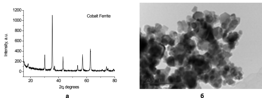
Фигура 1. Рентгенопорова дифрактограма на \text{CoFe}_2\text{O}_4 , получен чрез зол-гел метод (а) и ТЕМ-изображение на същата проба (б)
