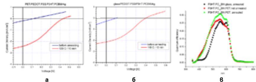
Фигура 1. V-A х-ки на светло на неотгрят и отгрят при температура 110-120°C фотоелемент върху (а) PET субстрат, (б) стъклен субстрат, както и (в) спектрите на квантова ефективност на ПОФ върху двата материала.
