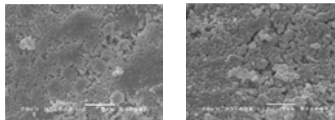
Фигура 1. СЕМ изображения на таблетки нагледени при 900 °C за 40 ч поглед отгоре: \text{LaCo}_{0.9}\text{Ni}_{0.1}\text{Fe}_{0.1}\text{O}_{3+\delta} (ляво) получен при обикновено налягане и (дясно) проба получена под високо кислородно налягане \text{LaCo}_{0.8}\text{Ni}_{0.1}\text{Fe}_{0.1}\text{O}_{3+\delta} .
