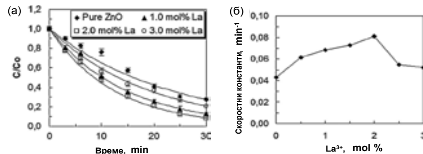
Фигура 1. Фотокаталитична активност на ZnO модифициран с различна La концентрация (а) и скоростни константи на фотокатализа (б). Началната концентрация на Реактивно Черно 5 е 20 ppm.
