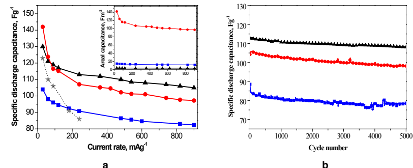
Фигура 1. Специфичен разряден капацитет като функция от токовото натоварване (а) и броя цикли при токово натоварване 240 \text{ mA g}^{-1} (б): ▲ – \alpha\beta\text{-Ni(OH)}_2 , ● – \text{NaNi}_{0.5}\text{Mn}_{0.5}\text{PO}_4 , ■ – \text{LiNi}_{0.5}\text{Mn}_{0.5}\text{PO}_4 ; * – симетричен
