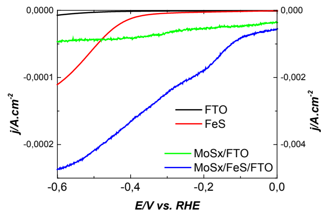
Фигура 2. Потенциодинамични криви на FTO, \text{FeSe} , \text{MoS}_x/\text{FTO} , и \text{MoS}_x/\text{FeS}/\text{FTO} в 0.2 \text{ M Na}_2\text{SO}_4 при облъчване със светлина 1 sun
