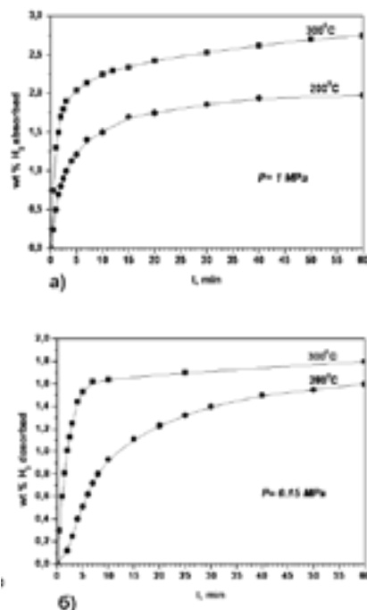
Фигура 1. Кинетични криви на : а) абсорбция на водород и б) десорбция на Mg_{2.1}Ni_{0.7}V_{0.3} – 5 мас. % активен въглен от кайсиеви костилки.
