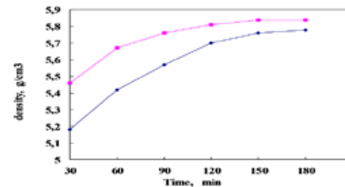
Фигура 2. Плътност на синтезираната керамика: ■ – при 1380^\circ C , ♦ – при 1300^\circ C
