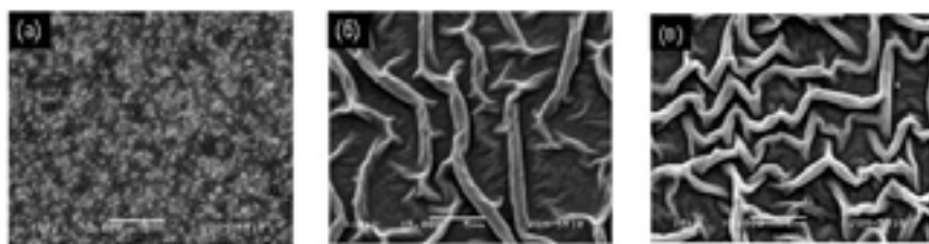
Фигура 1. SEM изображения на ZnO филми, получени върху стъклени подложки при различни температури на наляване: (а) 100 °С, (б) 300 °С и (в) 500 °С. Схематично представяне на активната повърхностна фотокаталитичните филми (г).
