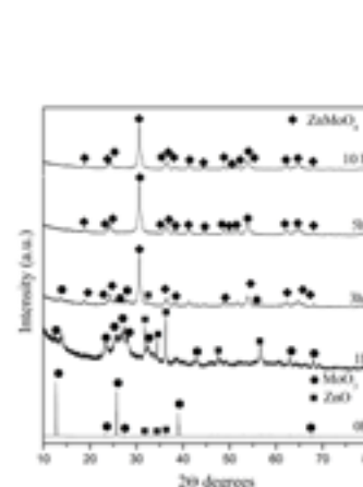
Фигура 1. Рентгенови дифрактограми на смес от \text{ZnO} и \text{MoO}_3 при скорост на активиране 850 об/мин.
